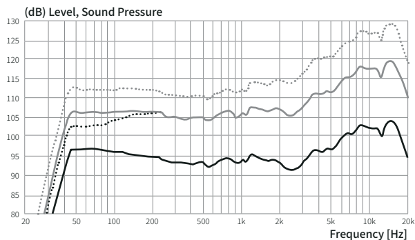
图 53. S12 PRO 低音音箱和 M-F3A PRO 音箱在不同组合方式下获得的频响
